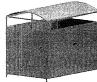
Контейнерная площадка 2-х местная (профлист) Размер (LxBxH, м) 2,53x1,56x2,18
